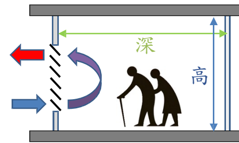
單面通風(深度不多於2倍高度)
